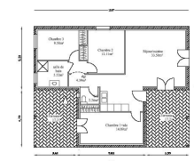
Plan rez de chaussée échelle : 1/100
