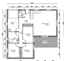
Plan rez de chaussée échelle : 1/100
